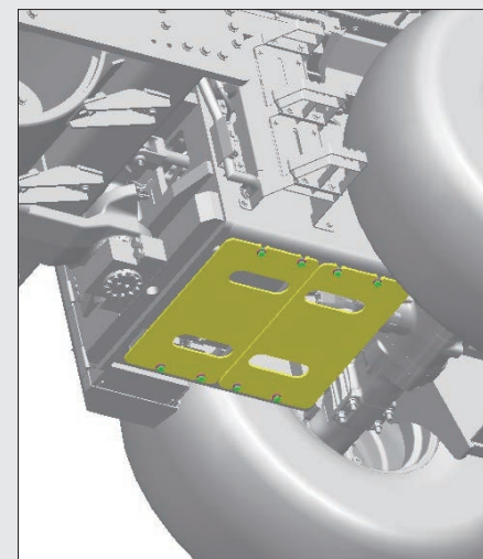
アンダーガード
